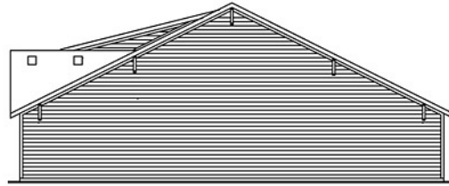
Right Elevation
